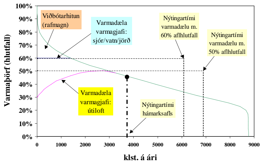
Mynd 1 Langæisferill varmaþarfar á SV-horni landsins. Hluttur varmadælu a) með útiloft og b) með sjó/vatn/jarðhita sem varmagjafa. Toppafl með öðrum orkugjafa t.d. rafmagni.
